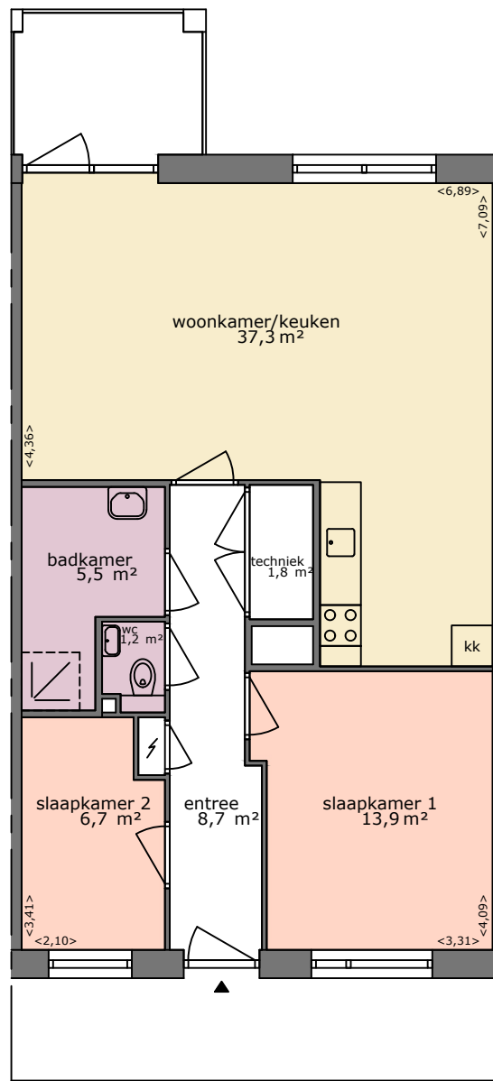
begane grond
