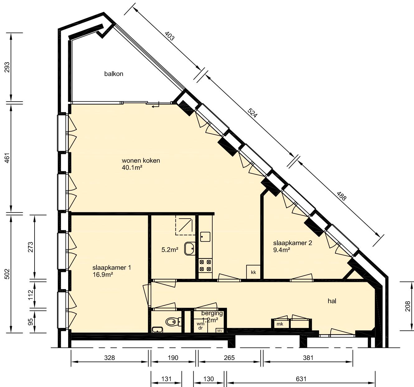
■ gebruiksooppervlak woonfunctie 94.72m 2 3e verdieping
