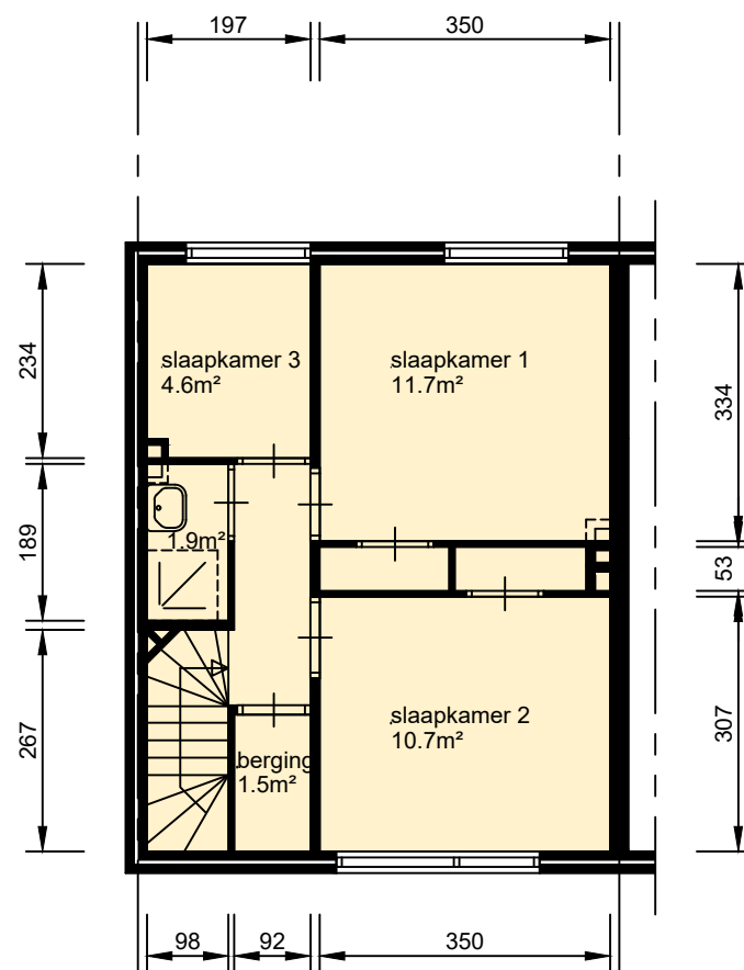
verdieping
