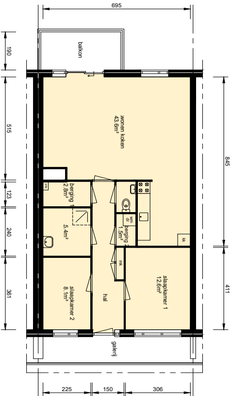
verdieping gebruiksovervlak woonruimte 87.46m 2
