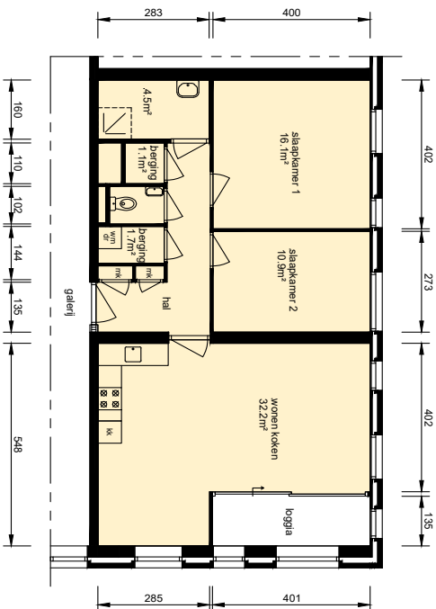
verdieping gebuiksoppervlak woofunctie 87.34m²
