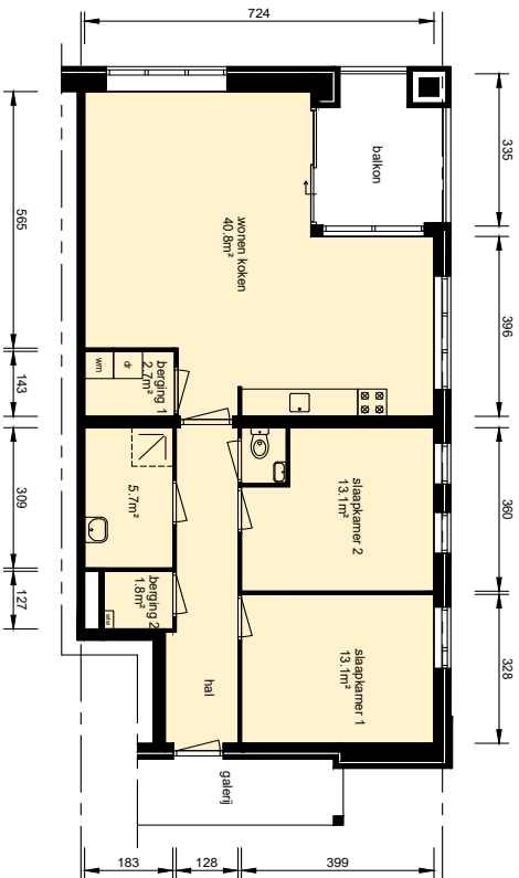
verdieping ■ gebruiksooppervlak woonfunctie 91.25m 2
