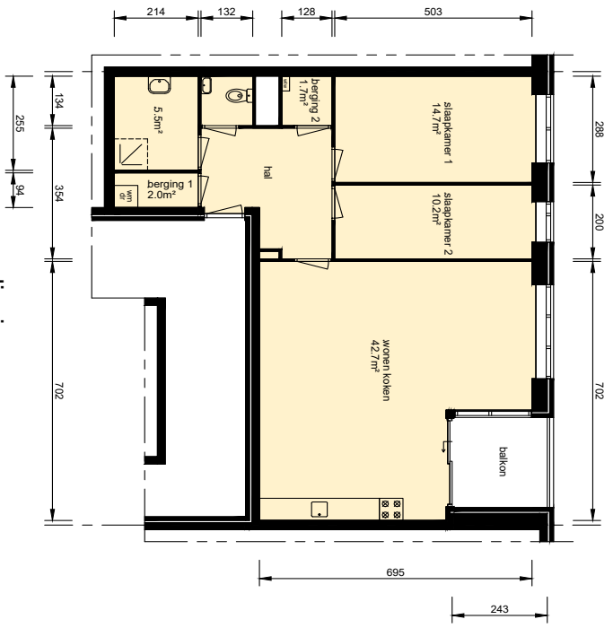
verdieping gebuiksoppendek woonruimte 90,14m 2
